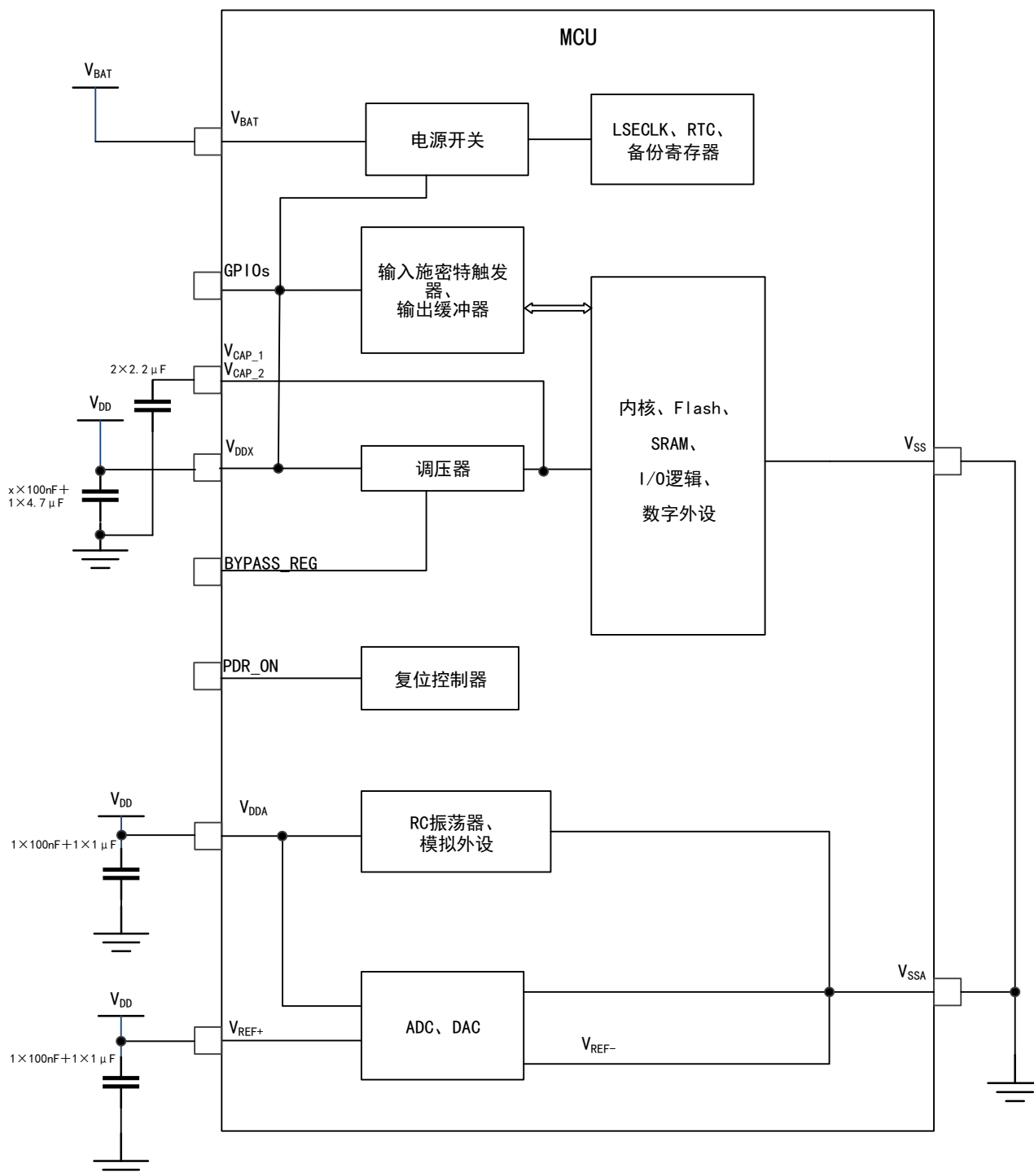
图 8 电源方案
