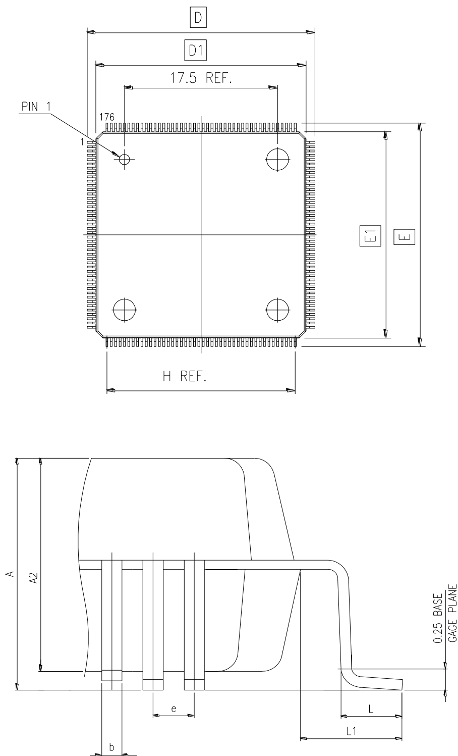
图 17 LQFP176 封装图
