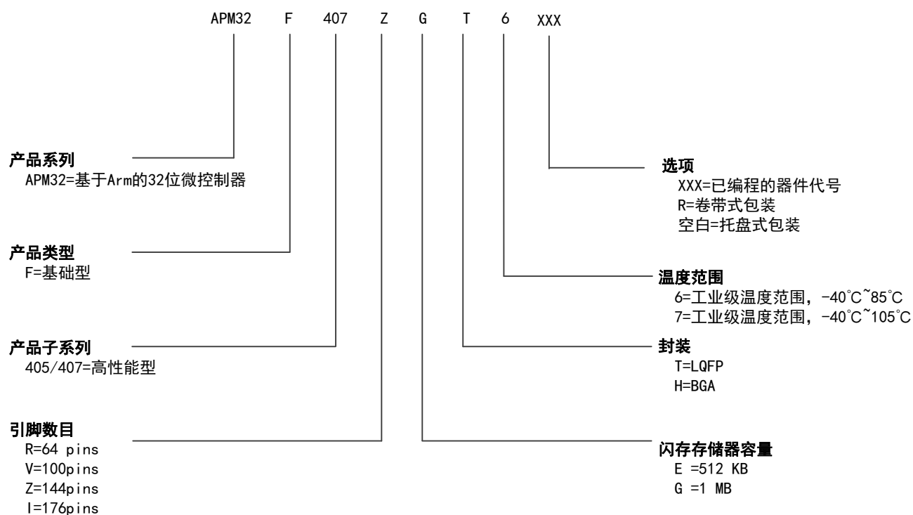
图 34 APM32F405xG 407xExG 系列订货信息图
