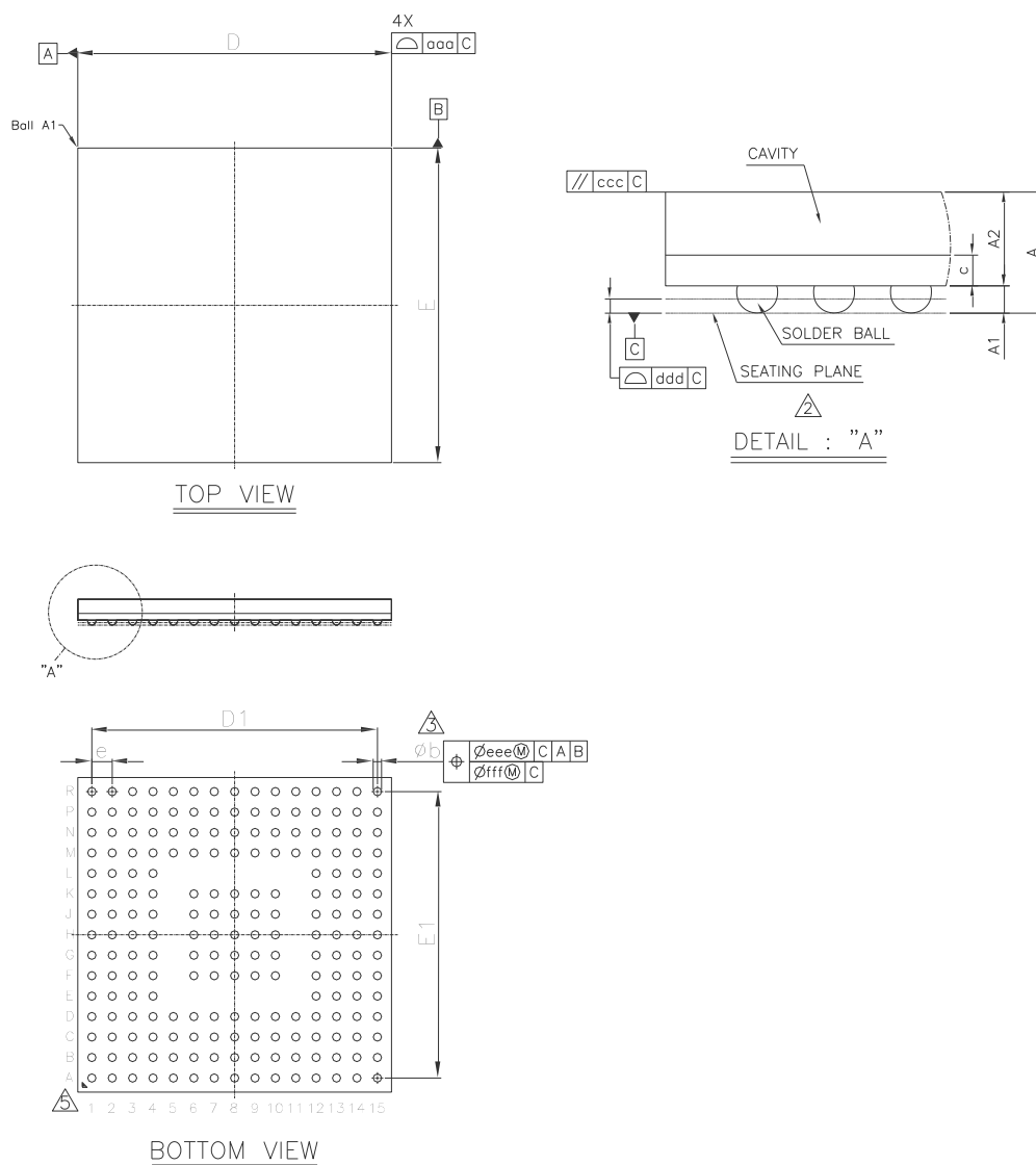
图 29 BGA176+25 封装图
